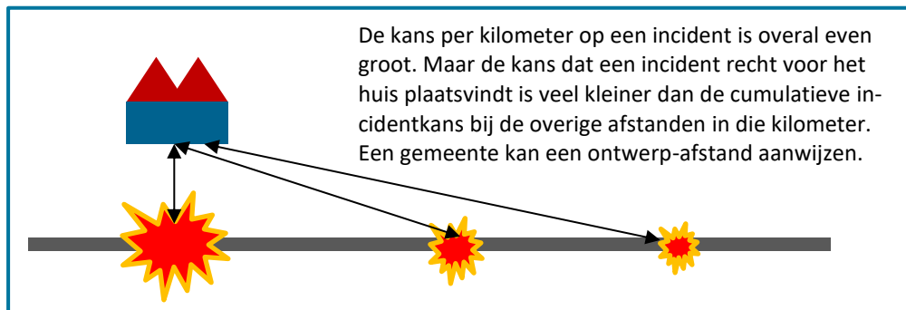
Figuur 5.1: Uitgaan van de kortste afstand of van een vastgestelde ontwerpafstand?
